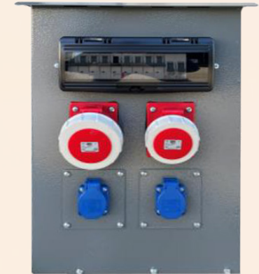
Bedienfeld „ISO Full Panel“
